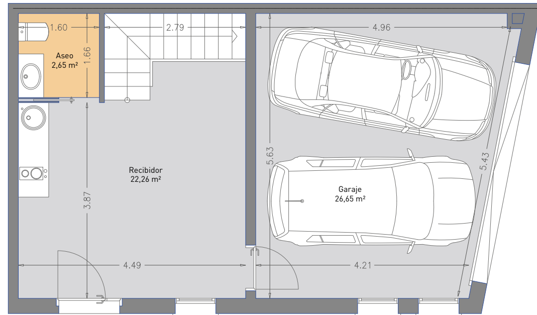
PLANTA BAJA
